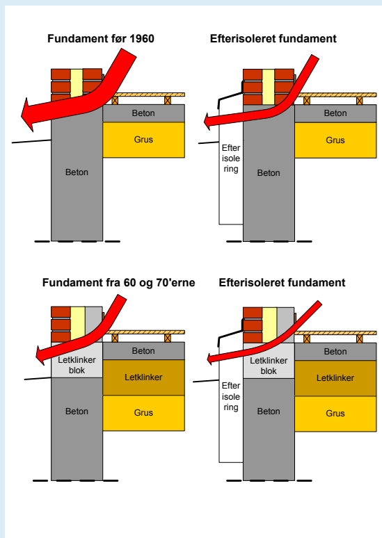
Efterisolering af sokkel/fundament.
