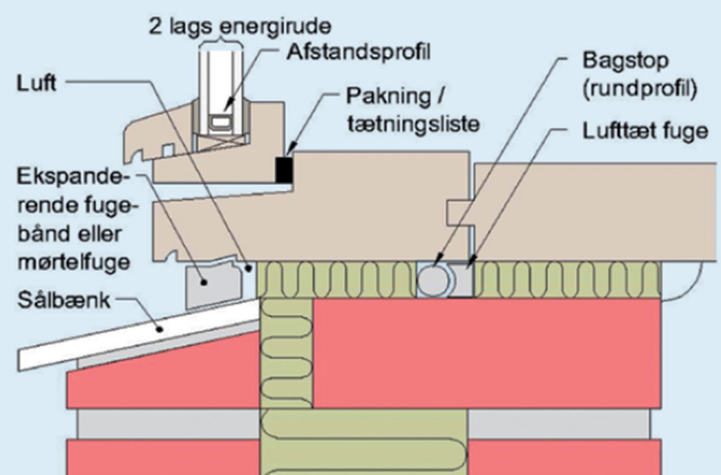
Vinduesfals med kuldebroisolering mellem for- og bagmur. Ny isolering mellem formur og bagmur.
