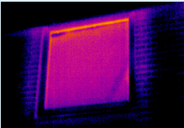
Termografisk billede af samling ved vindue. Set indefra. Der er størst varmetab ved samling.
