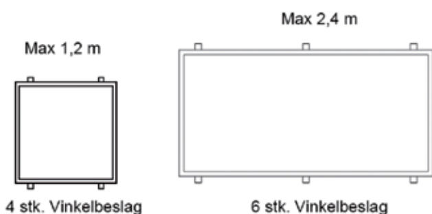
Figur 1: Fordeling af vinkelbeslag ved fastgørelse af ovenlys.
