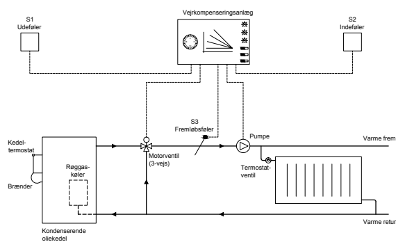
Figur 3. Olie- eller gasfuret kedelanlæg (med stort vandindhold)
