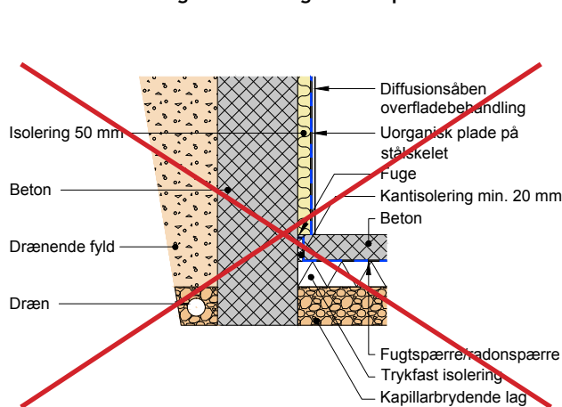
Kældervæg ved kældergulv med plade
