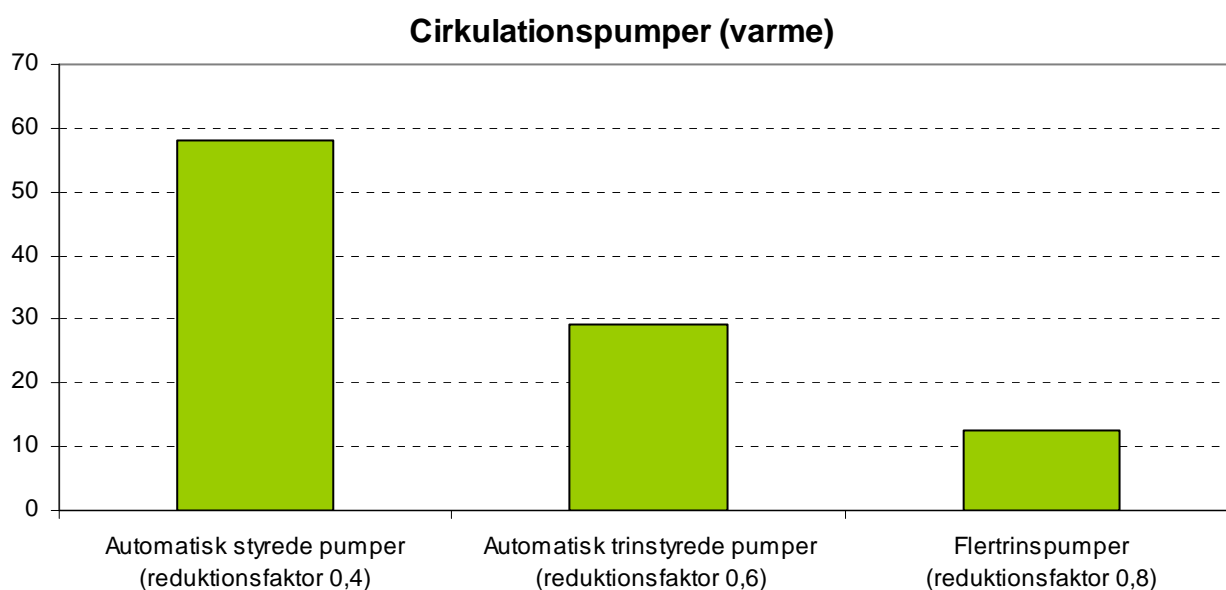
Figur 9 Fordeling af cirkulationspumpernes reduktionsfaktorer.
